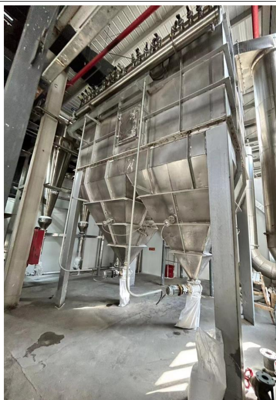
半纤生产线袋式除尘器
