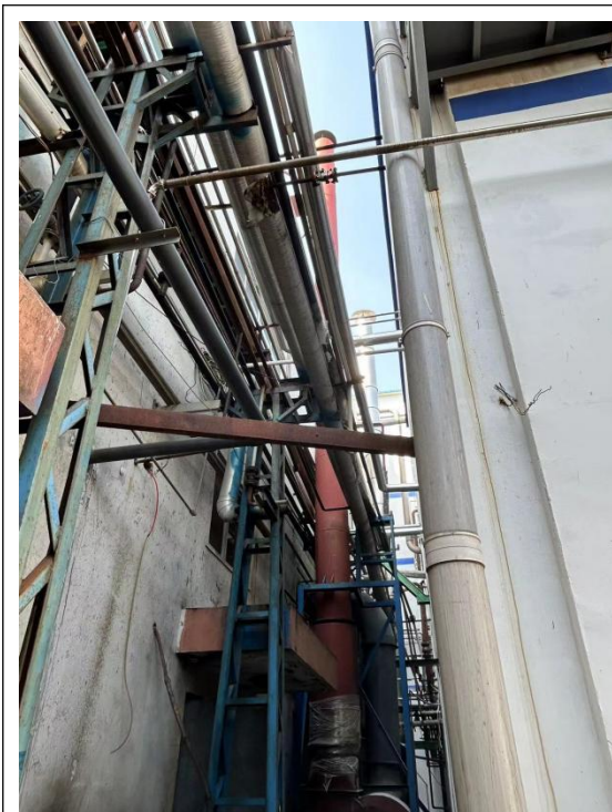
玉米芯干燥 2 套袋式+18m 排气管，红色排 气管老干燥，银色排气管新干燥
